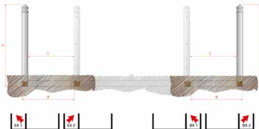
SOLUZIONE SX vista esterna
